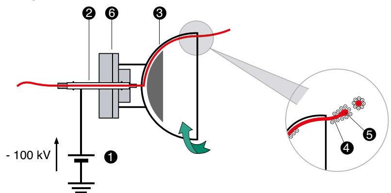
Bol tournant à haute vitesse de 5000 à 45000 tr./min en charge
